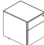
Art. MT2C Cassettiera metallica su ruote, 2 cassetti L42 x P54 x H54
